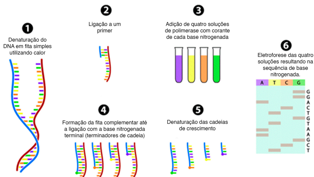
Figura 2. Principais aspectos do sequenciamento Sanger.
