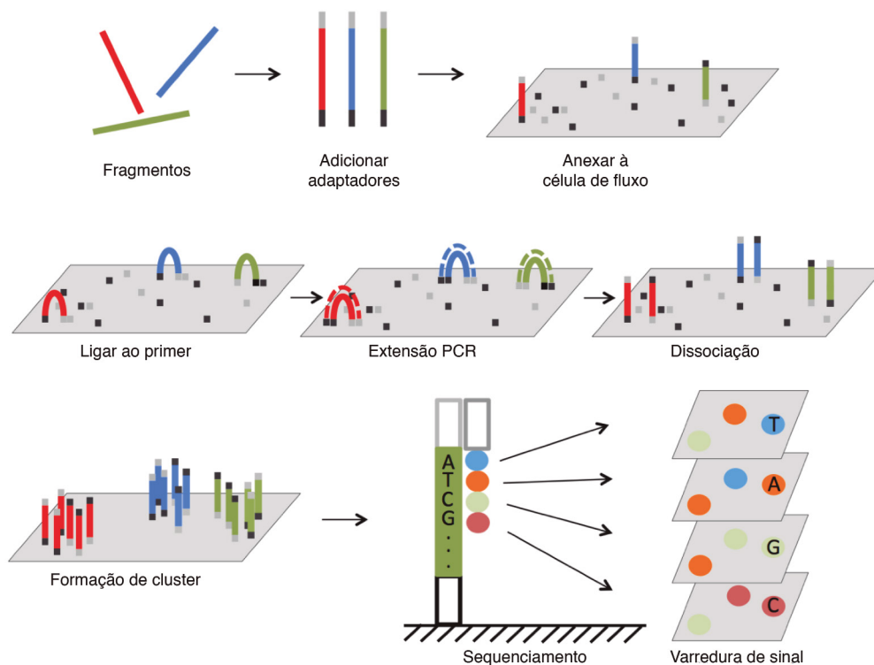
Figura 4. Esquema do processo de sequenciamento pelo método Illumina. Adaptado de Lu, Yuan, et al. 2016
